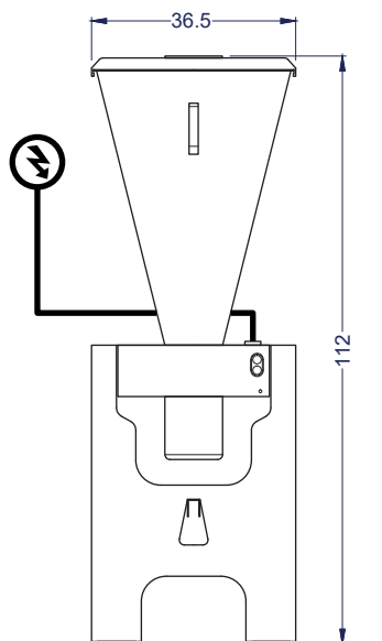
Vista Elevación
